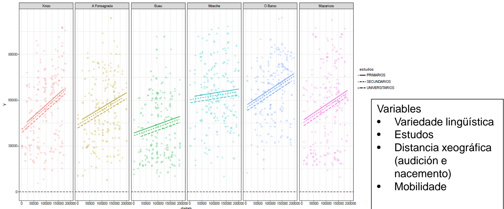
Figura 3: Modelo mixto axustado considerando o intercepto aleatorio e a pendente aleatoria por audición.
